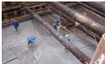
Baustelle - Kläranlage
